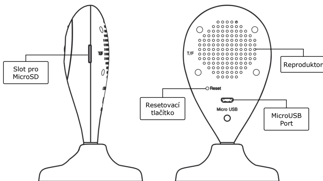
Obrázek 2 – Boční pohled a pohled zezadu
