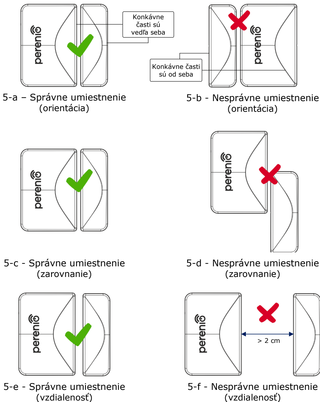
Obrázok 5 – Pravidlá inštalácie senzora a magnetu
