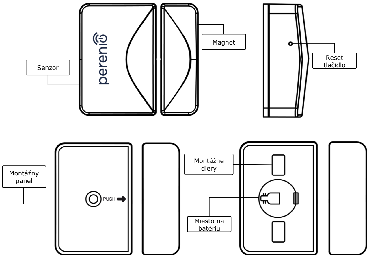
Obrázok 2 – Súčasti senzora otvorenia
