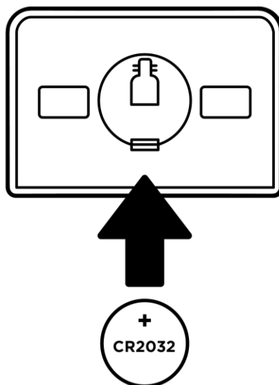
Obrázok 7 – Umiestnenie batérie v senzore otvorenia
